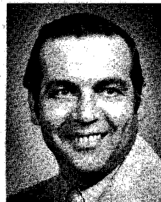
NORM POISSON
