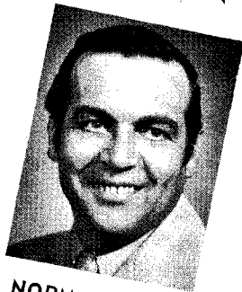
NORM POISSON
