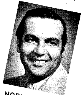
NORM POISSON
